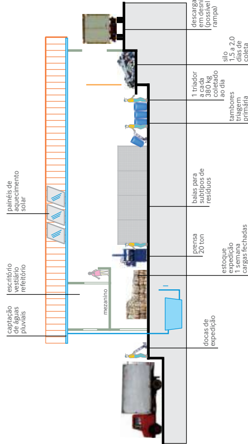
Figura 6 – Desenho ilustrativo do Galpão de Triagem de Resíduos Secos.
