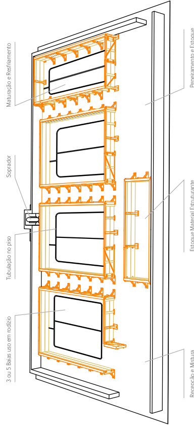
Figura 8 – Desenho ilustrativo do Galpão de Compostagem.
